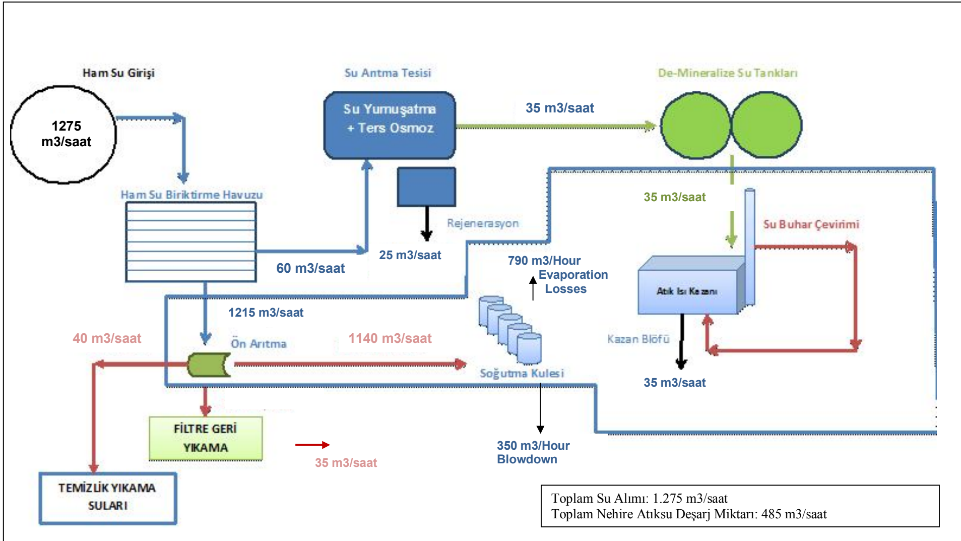
Şekil 62. Su Kütle Diyagramı
