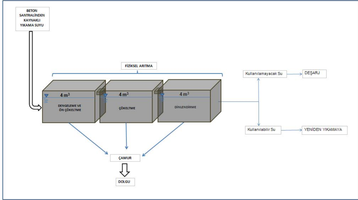
Şekil 56. Çökeltim Havuzu
