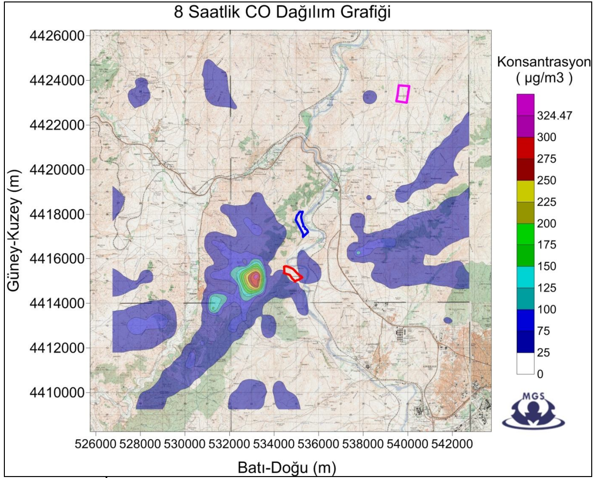
Şekil 77. İşletme Aşaması 8 Saatlik Karbon monoksit (CO) Emisyonu Dağılım Grafiği
