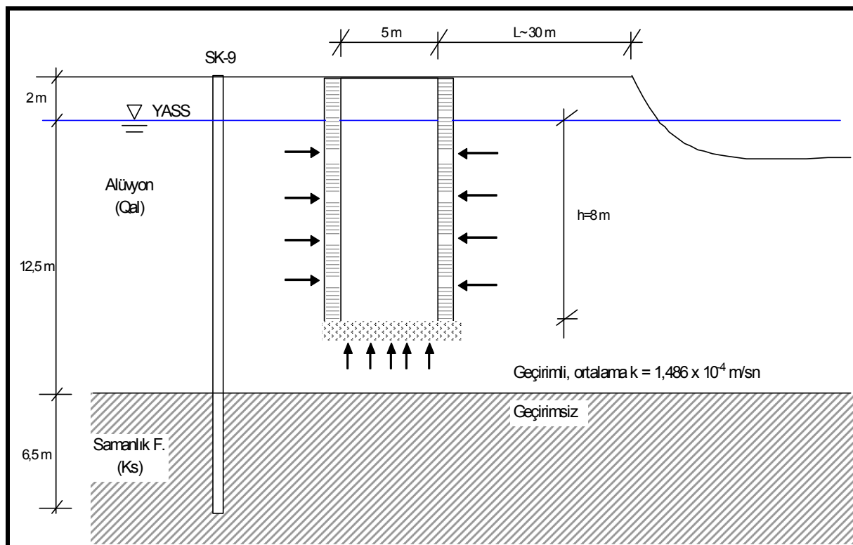
Şekil 37. SK-9 sondaj Lokasyonu Yakınında Açılacak Olan Keson Kuyunun Tahmini Ölçüleri ve Konumu
