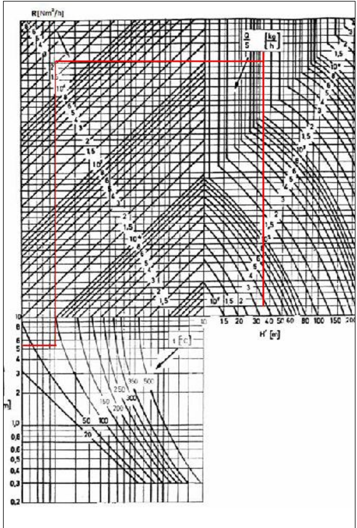
Şekil 81. NO 2 için Abak Hesabı
