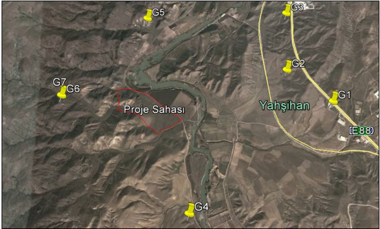
Şekil 50. Gürültü Ölçüm Noktalarını Gösterir Harita
