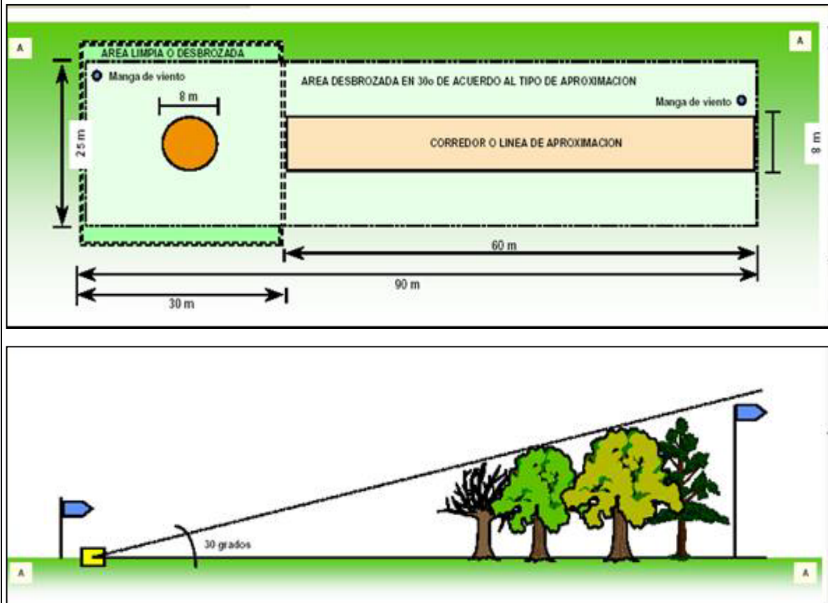
Figura 5-3. Dimensiones de helipuertos
