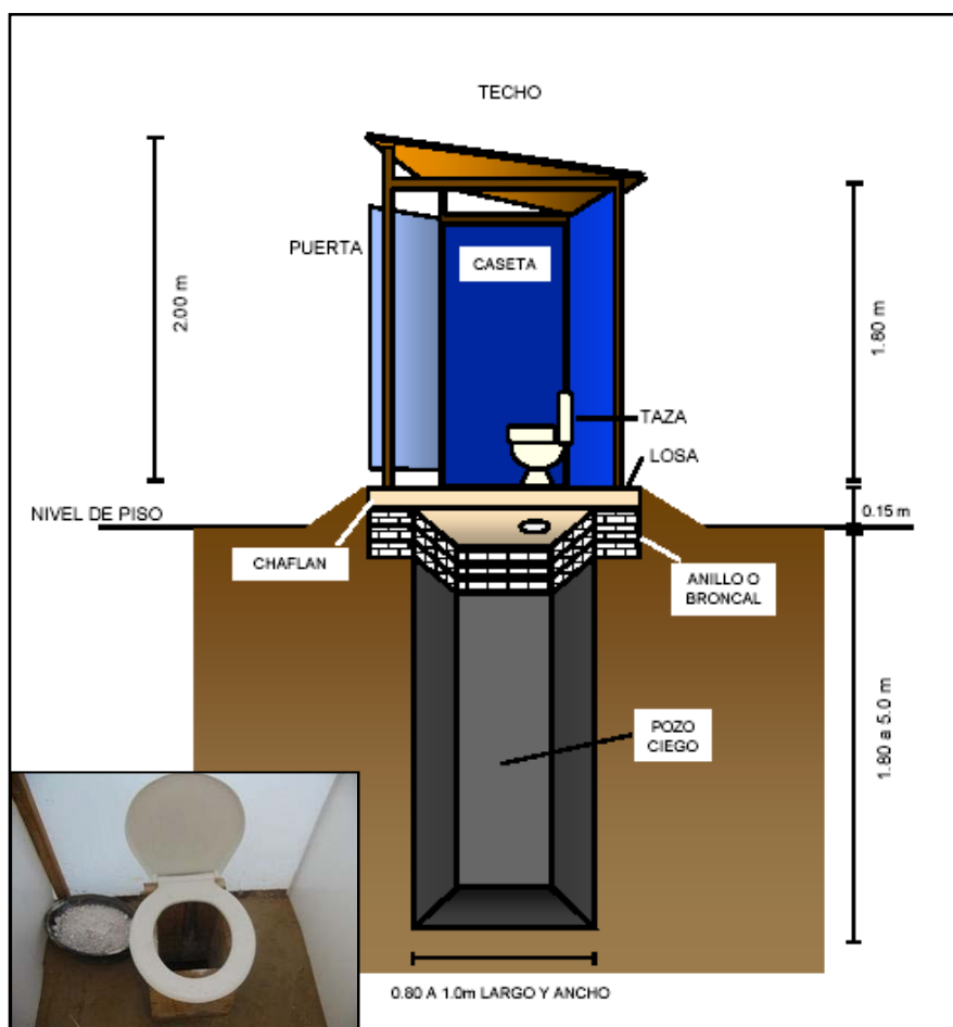
Figura 5-9 Letrina Sanitaria
