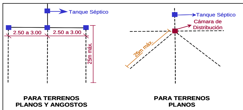
Figura 5-8. Disposiciones para campos de infiltración en terrenos planos
