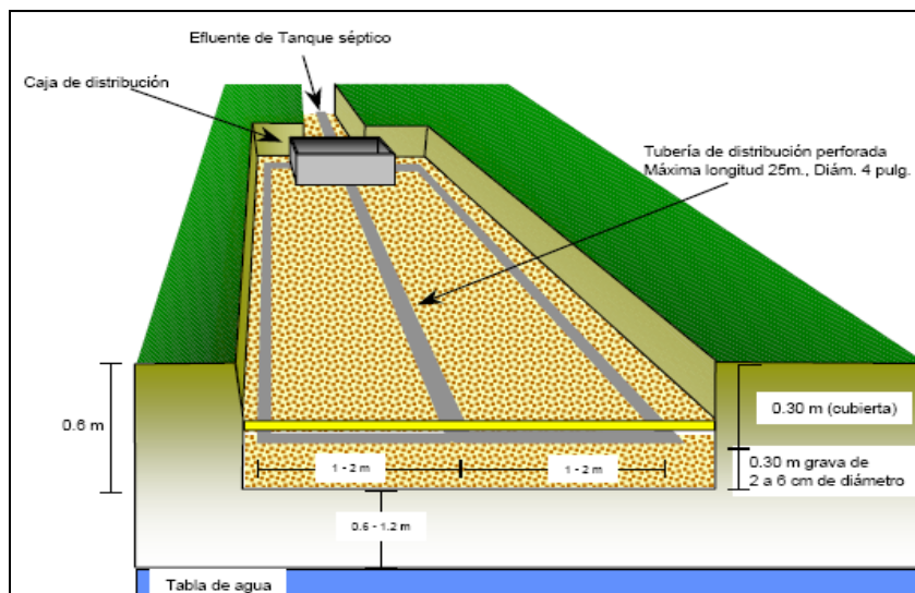
Figura 5-7 Campo de infiltración
