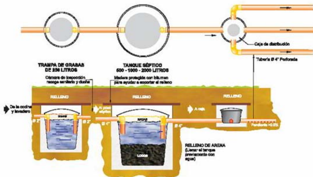
Figura 5-6. Sistema séptico
