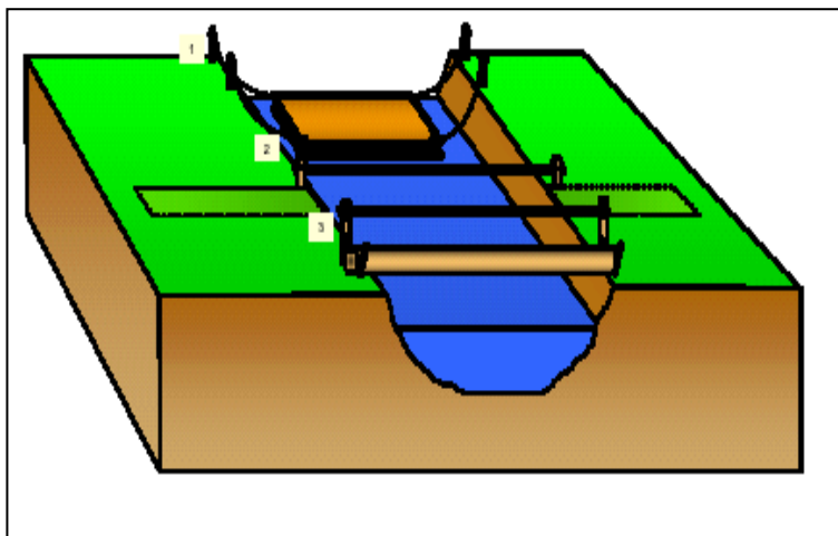
Figura 5-5. Modelo de cruces por cuerpos de agua
