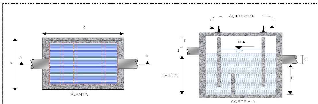
Figura 5-10. Diseño Tipo de la Trampa de Grasas para el Tratamiento de las Aguas Grises
