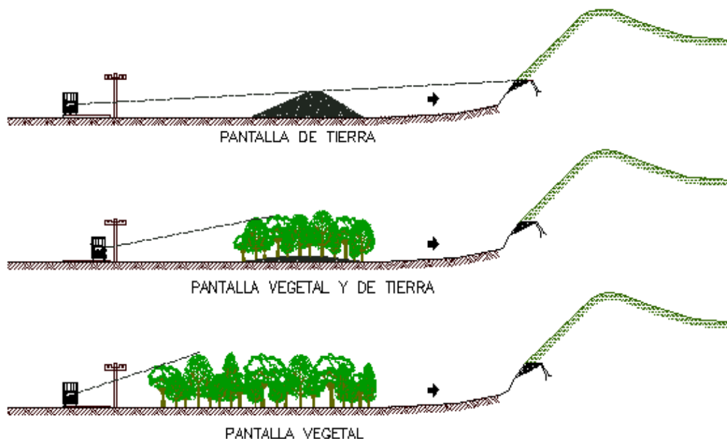
Figura 7-6. Pantallas tipo para ZODME
