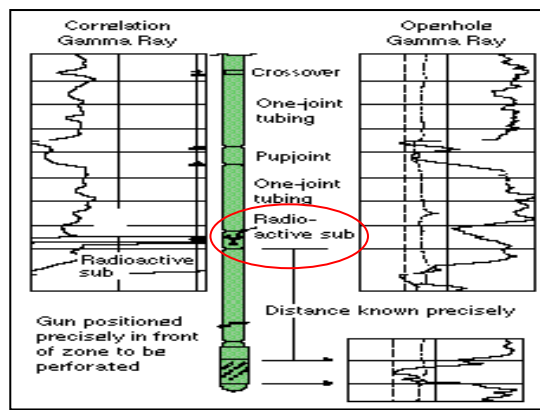
Figura 7-12. Localización de la fuente radiactiva en la sarta – Schlumberger
