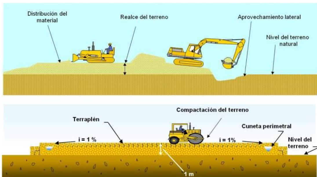
Figura 7-8. Préstamo lateral para la conformación de locaciones
