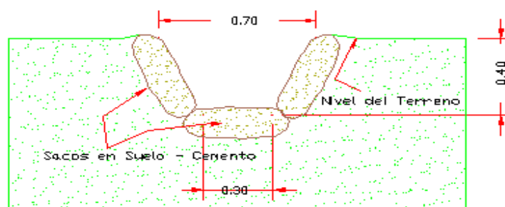
Figura 7-5. Sección de cunetas en sacos de suelo cemento en bermas intermedias.
