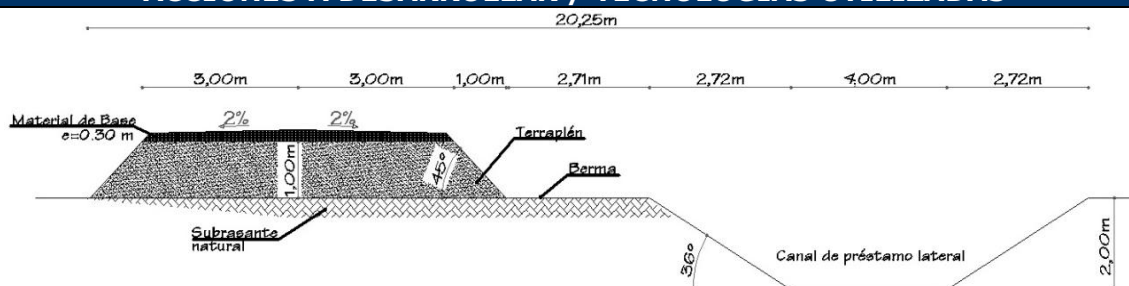
Figura 7-9. Sección transversal tipo del terraplén sobre tramos de vía de acceso a construir
