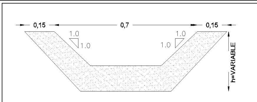
Figura 7-10. Diseño cuneta trapezoidal tipo
