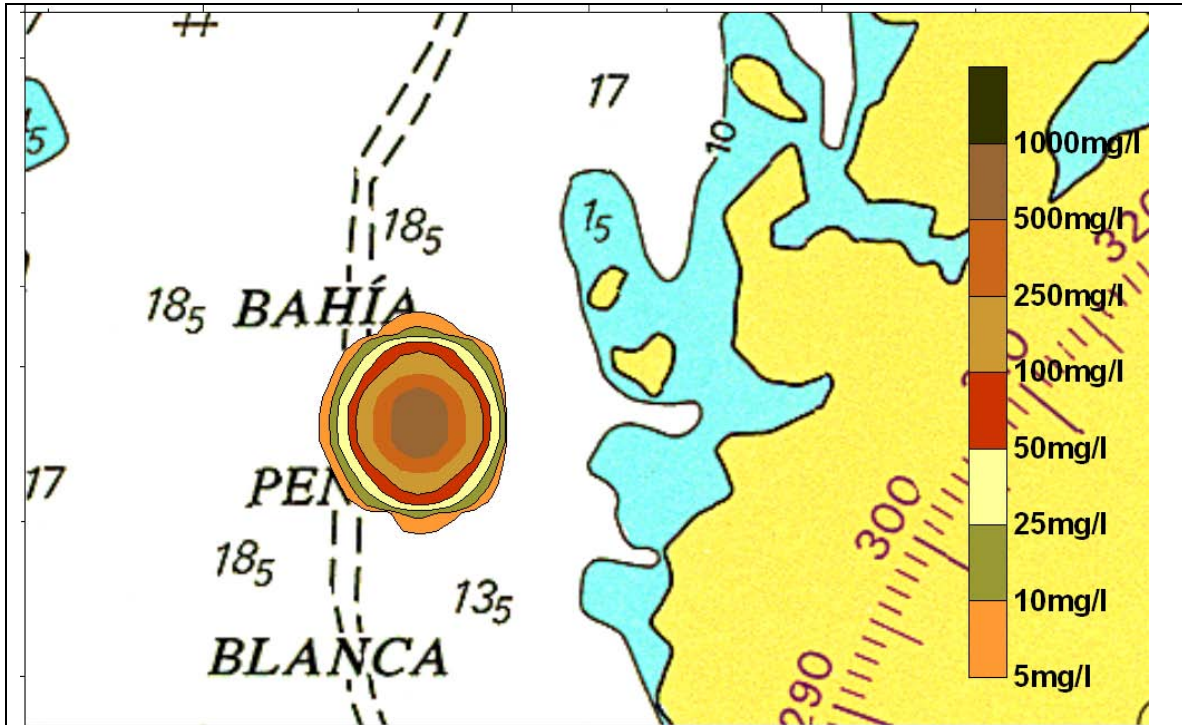
Figura 140 Escenario 11. Peña Blanca Oeste. Isolíneas de concentración a 6 m de profundidad, 1 hora después de la primera descarga.
