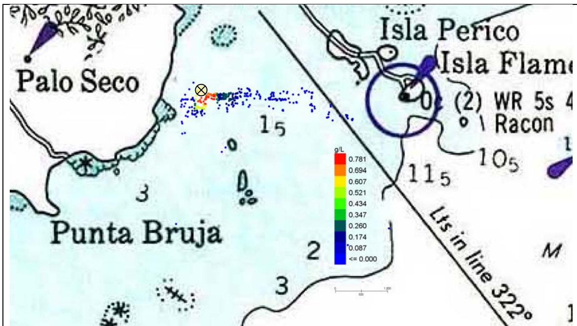
Figura 52 Escenario 4. Palo Seco. Detalle de las concentraciones de sólidos en la columna de agua a las 18 horas del comienzo del depósito.
