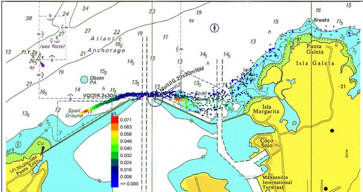
Figura 24 Escenario 2. Rompeolas Oeste. Detalle de las concentraciones de los sólidos en la columna de agua en el día 4 (96 horas) desde el comienzo del depósito.
