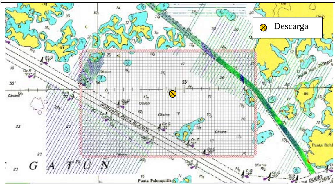
Figura 128 Malla de cálculo para la simulación de la evolución del sedimento en Peña Blanca Este.
