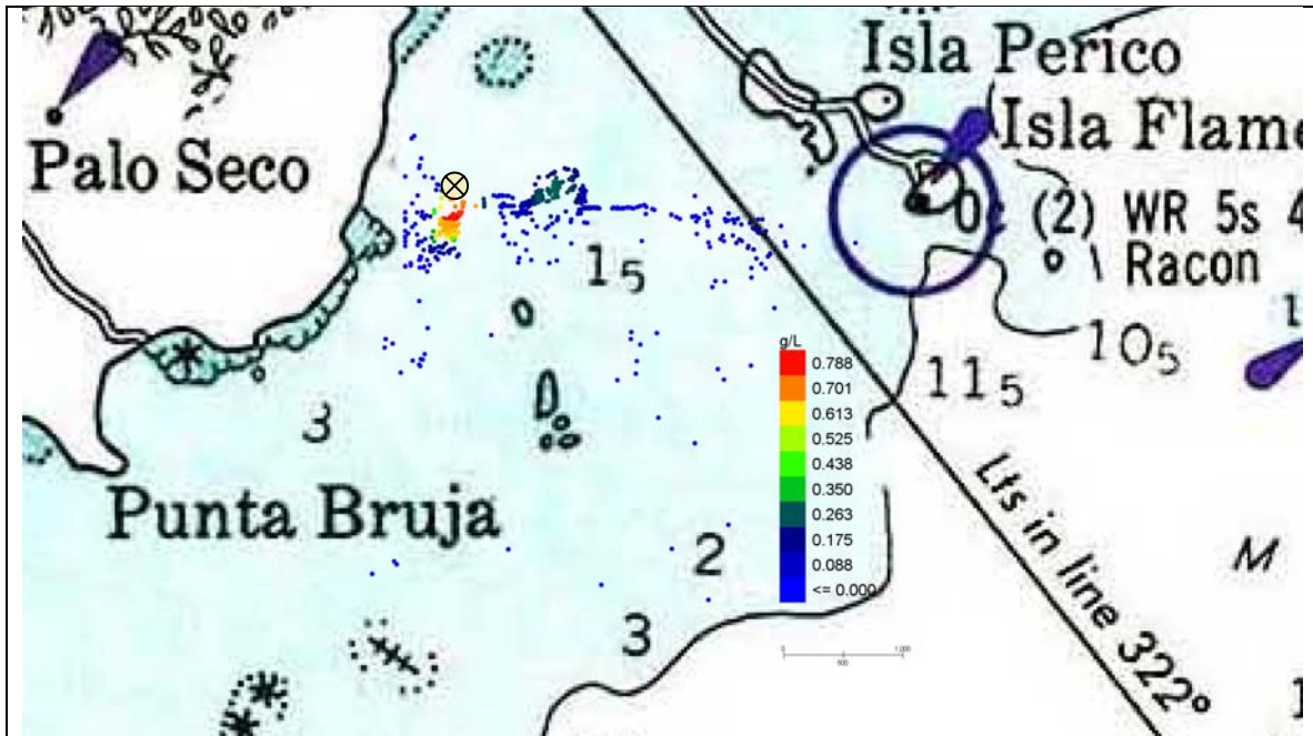
Figura 42 Escenario 3. Palo Seco. Detalle de las concentraciones de sólidos en la columna de agua en el día 2 (48 horas) desde el comienzo del depósito.
