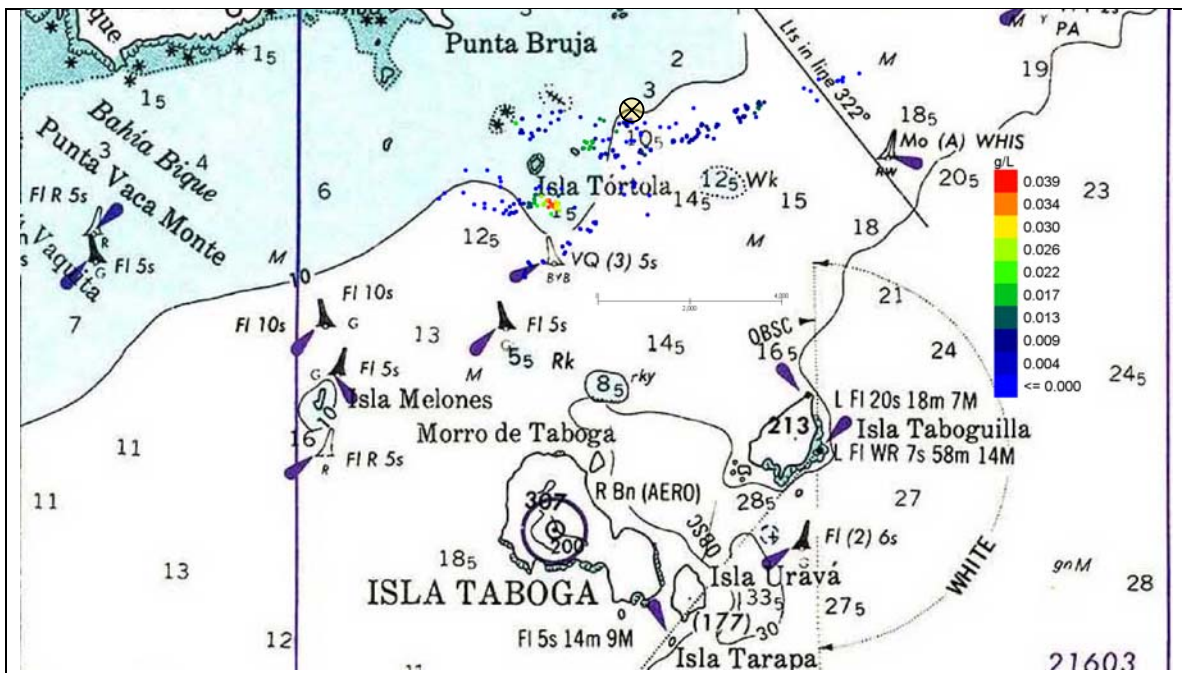
Figura 65 Escenario 5. Tortolita. Detalle de las concentraciones de sólidos en la columna de agua a las 12 horas del comienzo del depósito.
