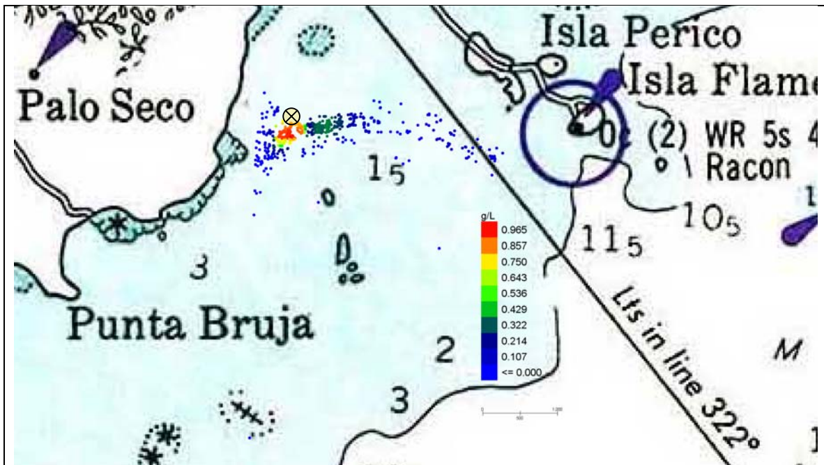
Figura 41 Escenario 3. Palo Seco. Detalle de las concentraciones de sólidos en la columna de agua en el día 1 (24 horas) desde el comienzo del depósito.
