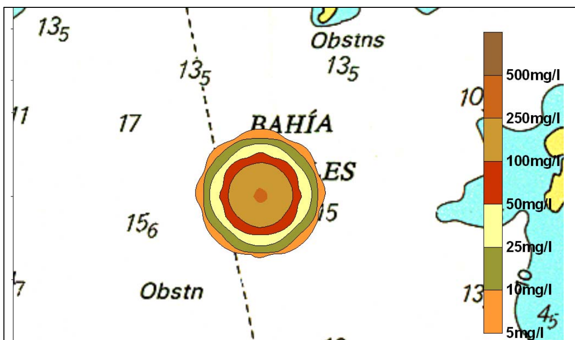
Figura 151 Escenario 12. Frijoles. Isolíneas de concentración a 6 m de profundidad, 2 horas después de la primera descarga
