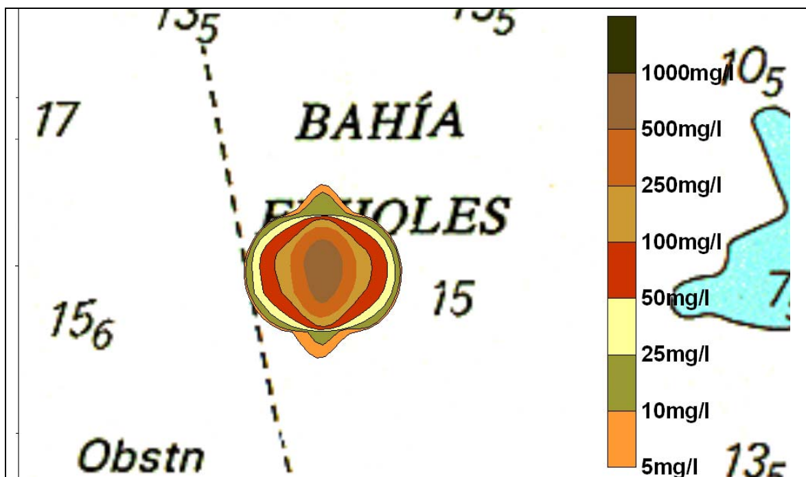
Figura 150 Escenario 12. Frijoles. Isolíneas de concentración a 6 m de profundidad, 1 hora después de la primera descarga.
