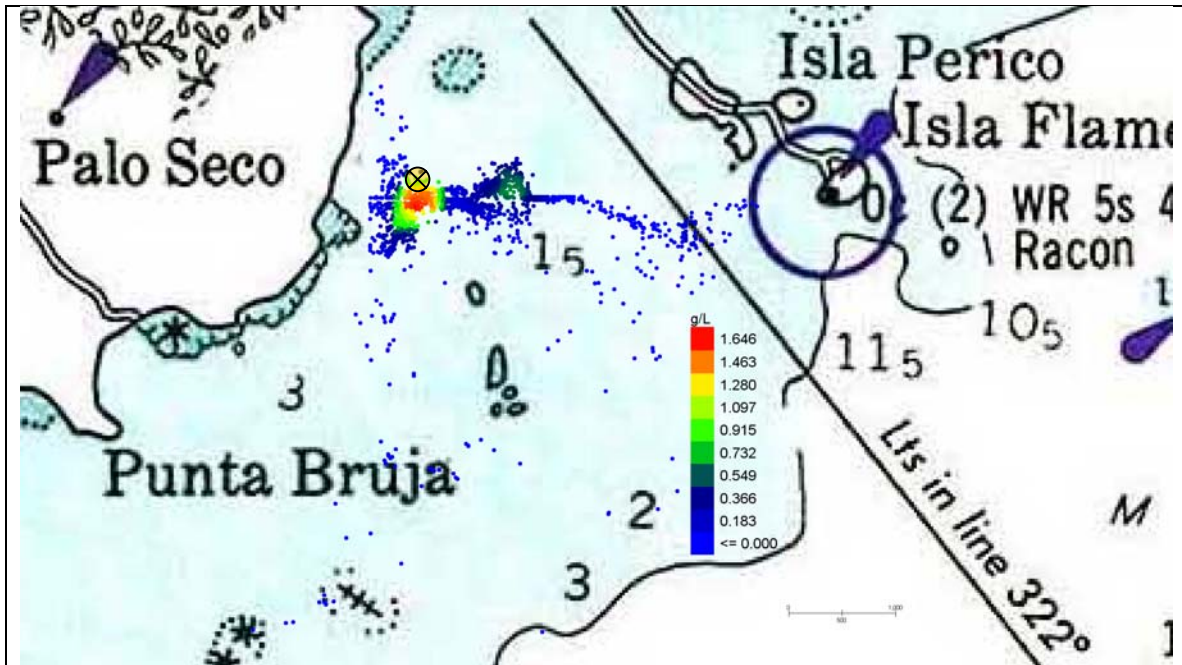
Figura 55 Escenario 4. Palo Seco. Detalle de las concentraciones de sólidos en la columna de agua en el día 3 (72 horas) desde el comienzo del depósito.
