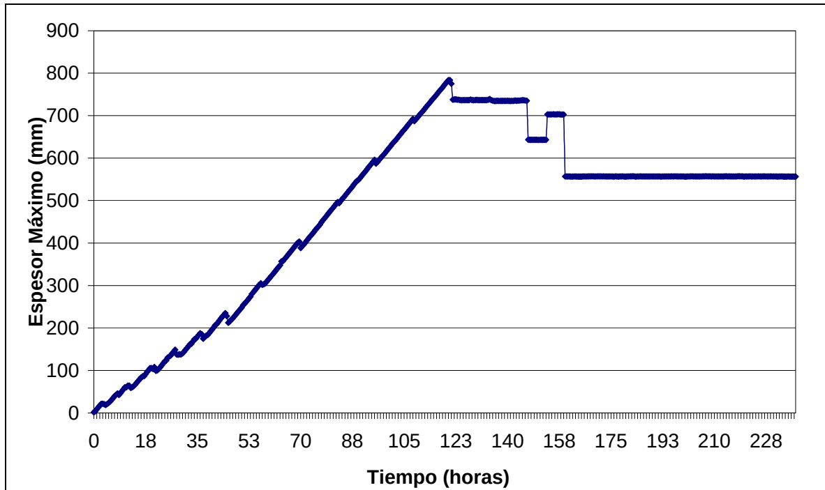
Figura 113 Escenario 8. Tortolita Sur. Espesores máximos del material depositado en el fondo.
