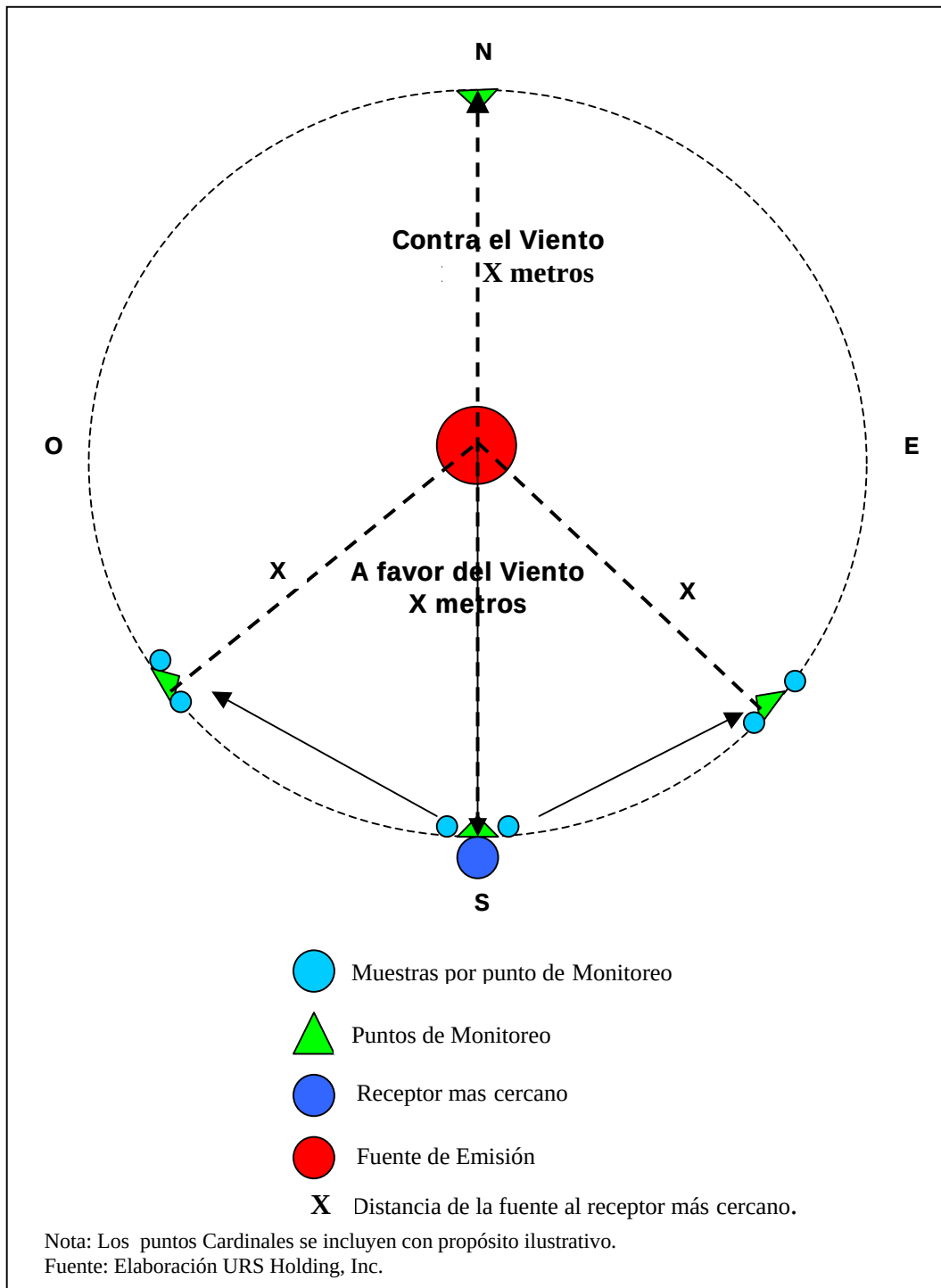
Figura A2-1 Esquema de Toma de Muestra por Fuente con Nasal Ranger
