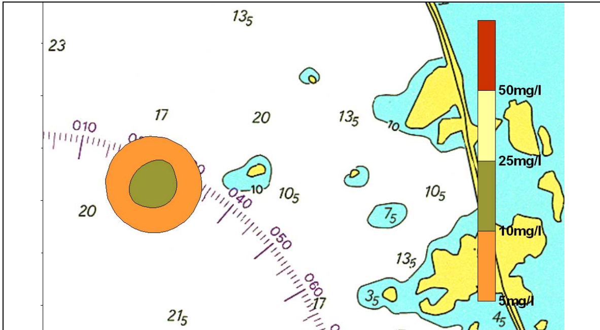
Figura 124 Escenario 9. Monte Lirio. Isolíneas de concentración a 3 m de profundidad, 8 horas después de la primera descarga.
