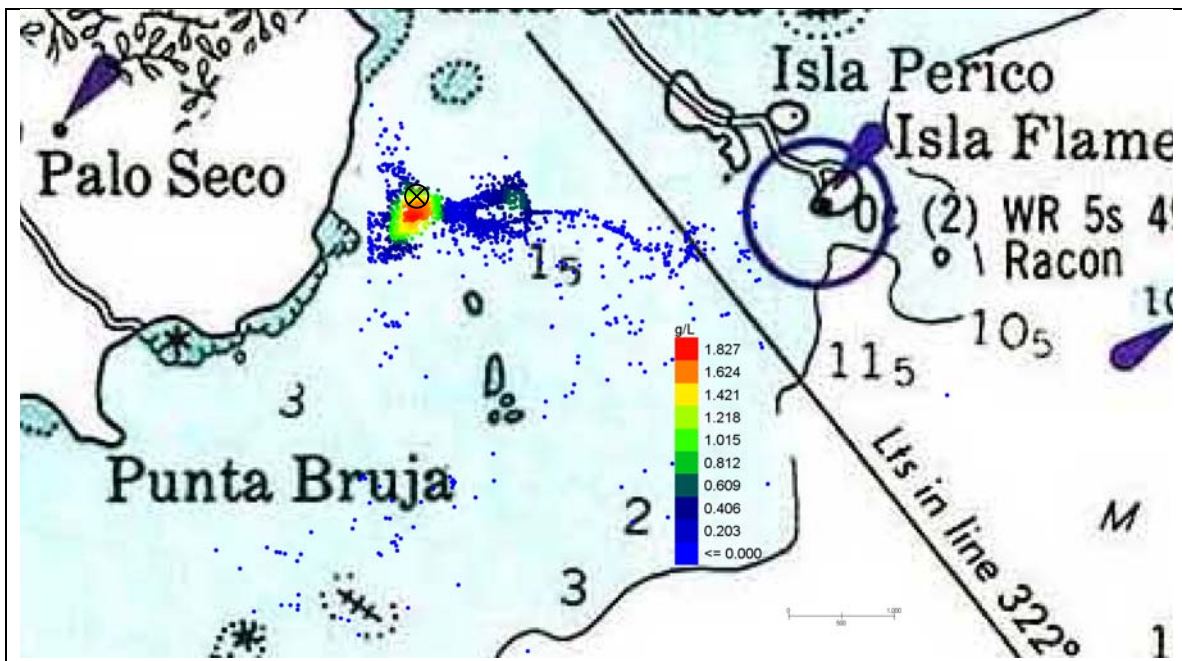
Figura 56 Escenario 4. Palo Seco. Detalle de las concentraciones de sólidos en la columna de agua en el día 4 (96 horas) desde el comienzo del depósito.
