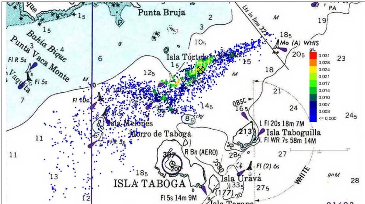
Figura 108 Escenario 8. Tortolita Sur. Detalle de las concentraciones de sólidos en la columna de agua en el día 4 (96 horas) desde el comienzo del depósito.
