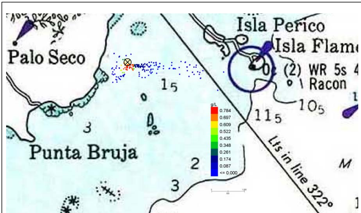
Figura 39 Escenario 3. Palo Seco. Detalle de las concentraciones de sólidos en la columna de agua a las 12 horas del comienzo del depósito.
