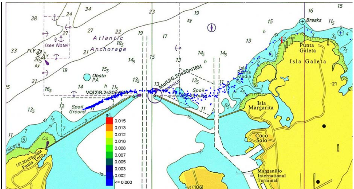
Figura 12 Escenario 1. Rompeolas Oeste. Detalle de las concentraciones de los sólidos en la columna de agua en el día 4 (96 horas) desde el comienzo del depósito.
