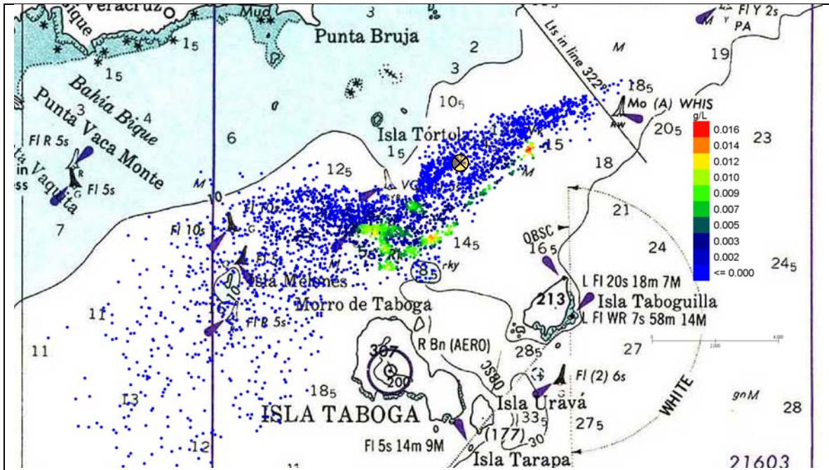
Figura 110 Escenario 8. Tortolita Sur. Detalle de las concentraciones de sólidos en la columna de agua en el día 6 (144 horas) desde el comienzo del depósito.
