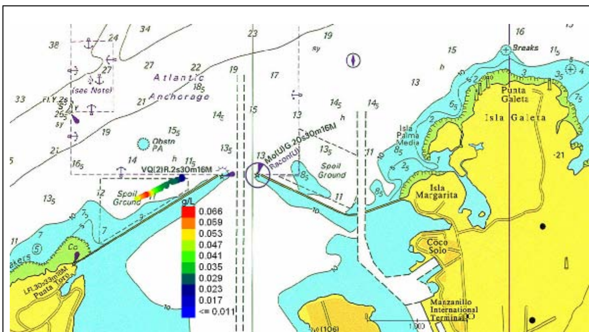
Figura 18 Escenario 2. Rompeolas Oeste. Detalle de las concentraciones de los sólidos en la columna de agua a las 6 horas desde el comienzo del depósito.
