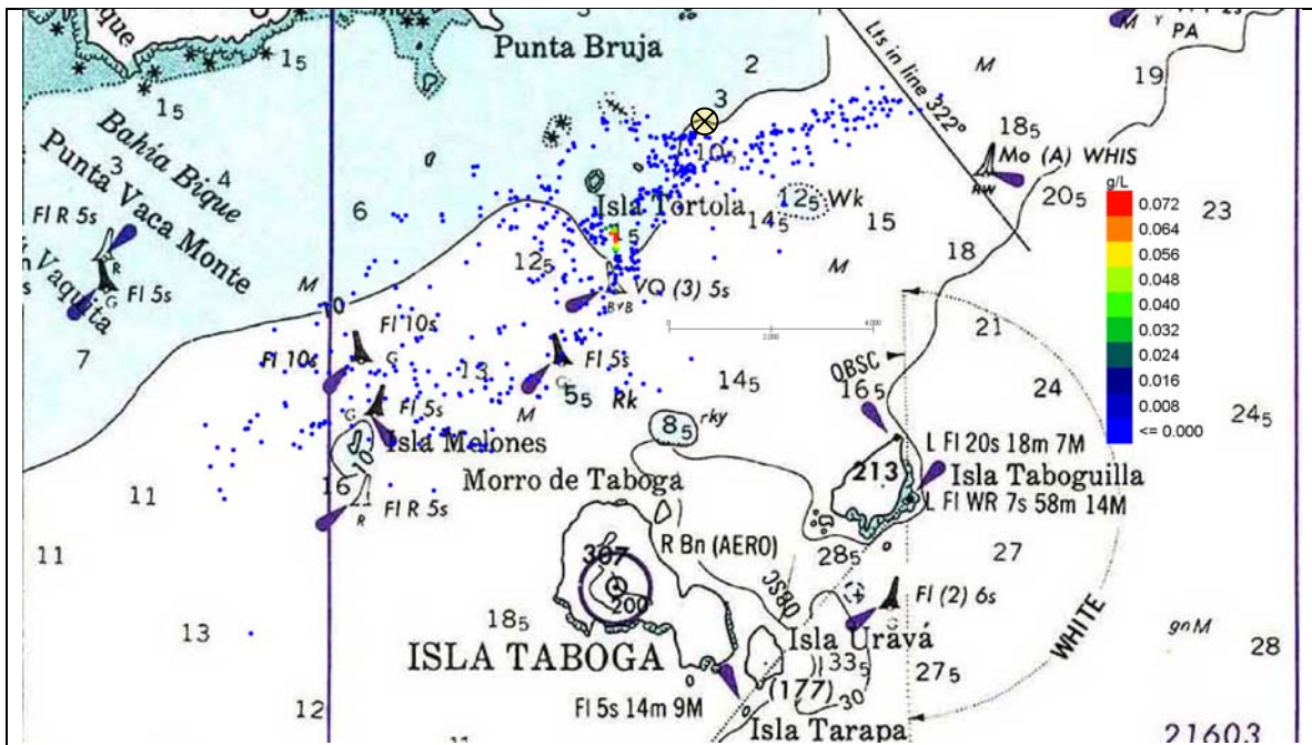
Figura 69 Escenario 5. Tortolita. Detalle de las concentraciones de sólidos en la columna de agua en el día 3 (72 horas) desde el comienzo del depósito.
