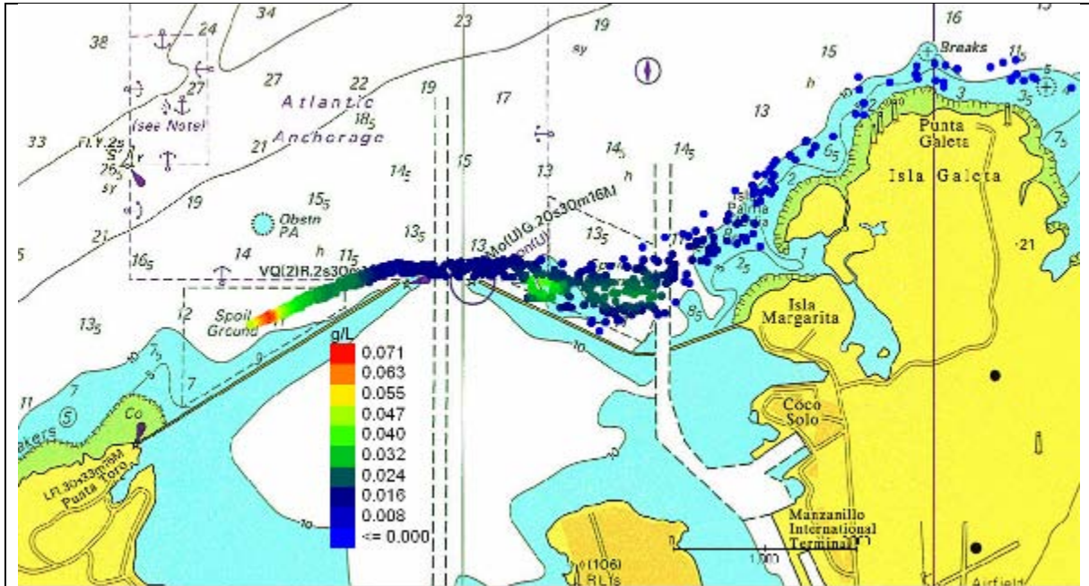
Figura 22 Escenario 2. Rompeolas Oeste. Detalle de las concentraciones de los sólidos en la columna de agua en el día 2 (48 horas) desde el comienzo del depósito.
