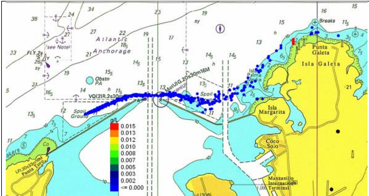
Figura 15 Escenario 1. Rompeolas Oeste. Detalle de las concentraciones de los sólidos en la columna de agua en el día 7 (168 horas) desde el comienzo del depósito
