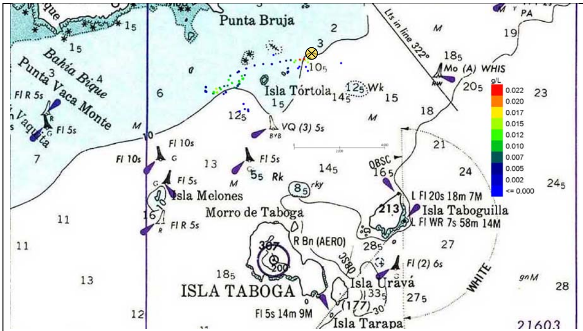
Figura 64 Escenario 5. Tortolita. Detalle de las concentraciones de sólidos en la columna de agua a las 6 horas del comienzo del depósito.
