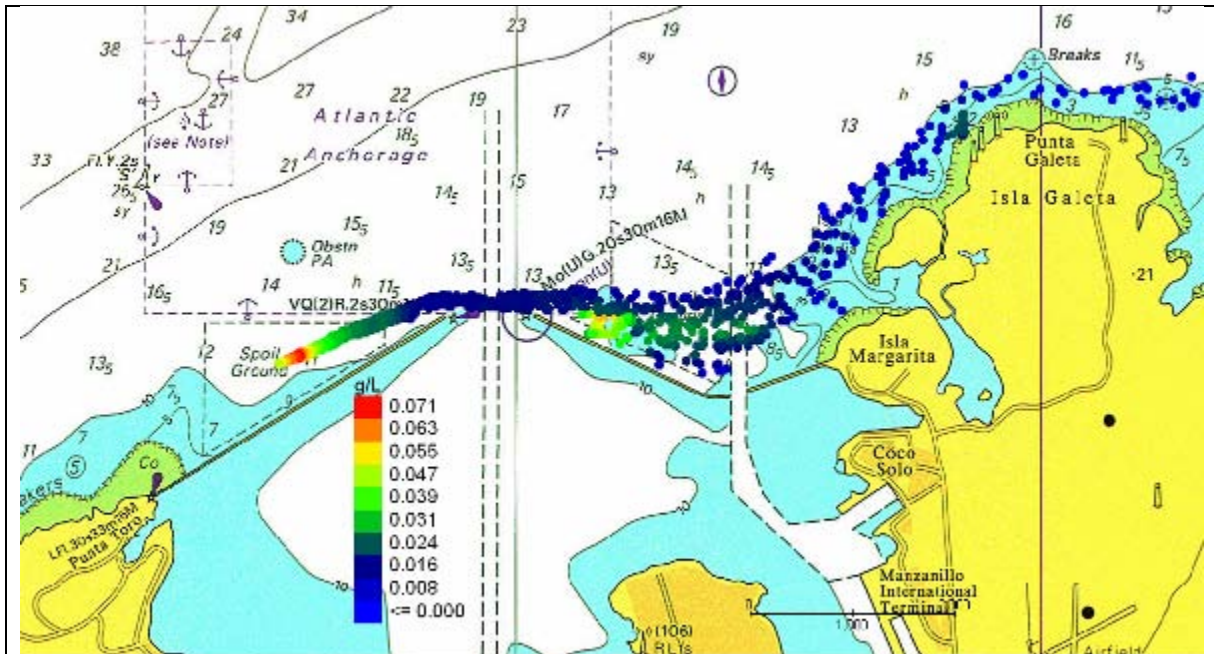
Figura 23 Escenario 2. Rompeolas Oeste. Detalle de las concentraciones de los sólidos en la columna de agua en el día 3 (72 horas) desde el comienzo del depósito.
