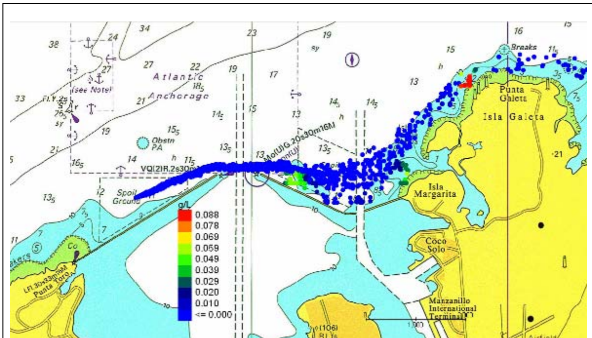
Figura 27 Escenario 1. Rompeolas Oeste. Detalle de las concentraciones de los sólidos en la columna de agua en el día 7 (168 horas) desde el comienzo del depósito.
