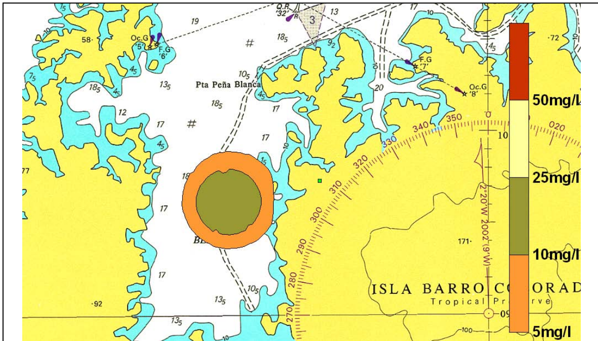
Figura 144 Escenario 11. Peña Blanca Oeste. Isolíneas de concentración a 6 m de profundidad, 8 horas después de la primera descarga.
