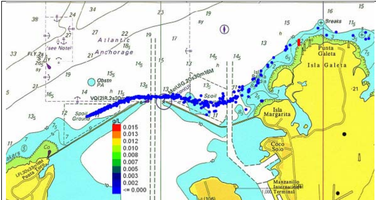
Figura 13 Escenario 1. Rompeolas Oeste. Detalle de las concentraciones de los sólidos en la columna de agua en el día 5 (120 horas) desde el comienzo del depósito
