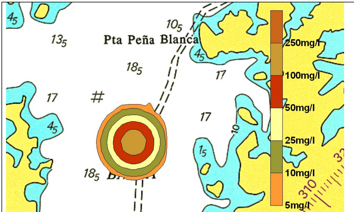
Figura 141 Escenario 11. Peña Blanca Oeste. Isolíneas de concentración a 6 m de profundidad, 2 horas después de la primera descarga.
