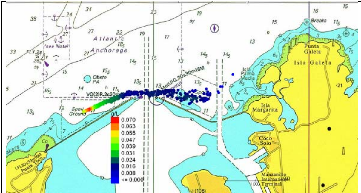
Figura 9 Escenario 1. Rompeolas Oeste. Detalle de las concentraciones de los sólidos en la columna de agua en el día 1 (24 horas) desde el comienzo del depósito.
