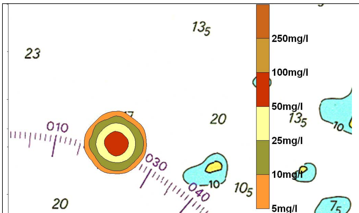
Figura 121 Escenario 9. Monte Lirio. Isolíneas de concentración a 3 m de profundidad, 2 horas después de la primera descarga.
