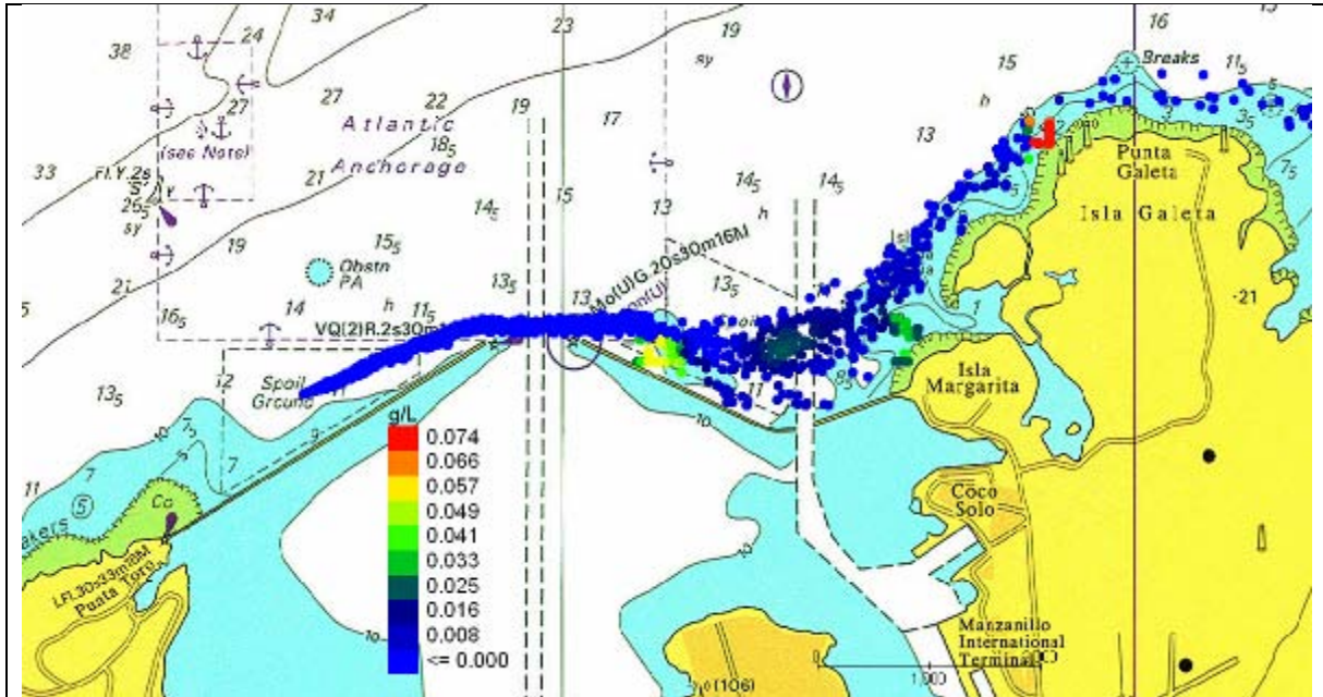
Figura 26 Escenario 2. Rompeolas Oeste. Detalle de las concentraciones de los sólidos en la columna de agua en el día 6 (144 horas) desde el comienzo del depósito.
