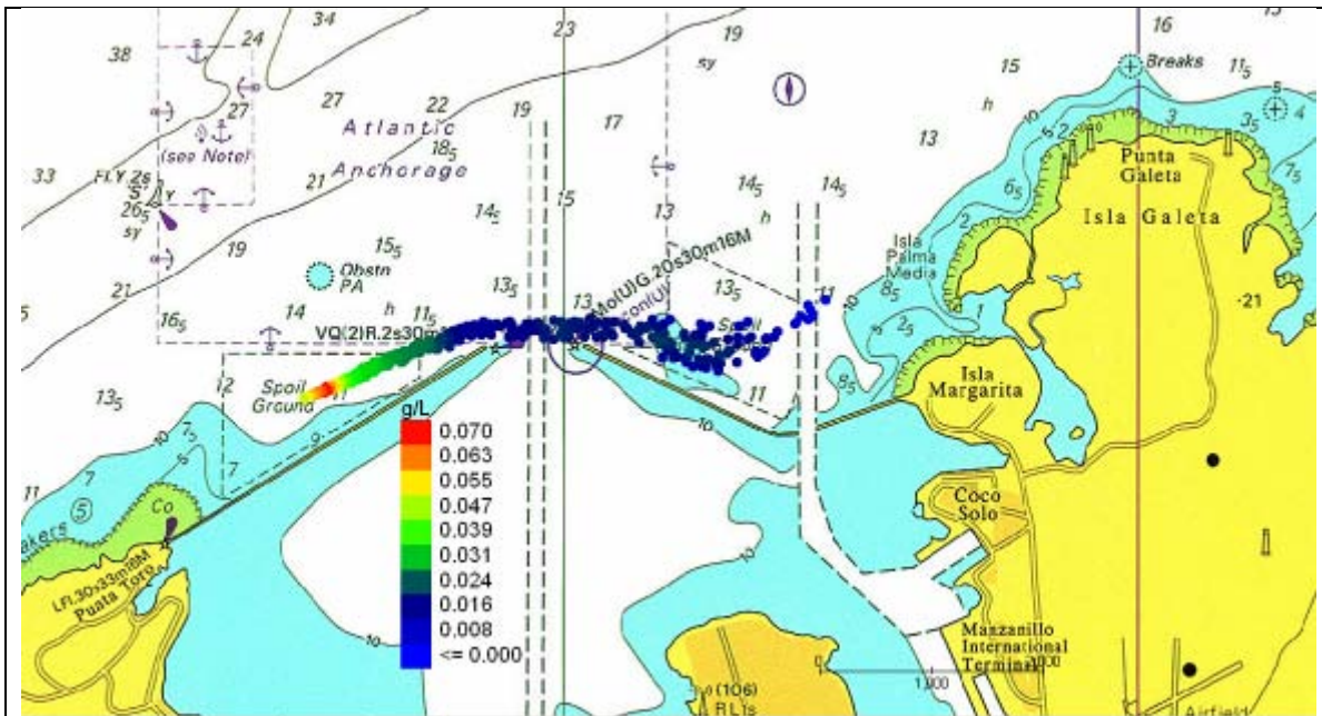
Figura 21 Escenario 2. Rompeolas Oeste. Detalle de las concentraciones de los sólidos en la columna de agua en el día 1 (24 horas) desde el comienzo del depósito.
