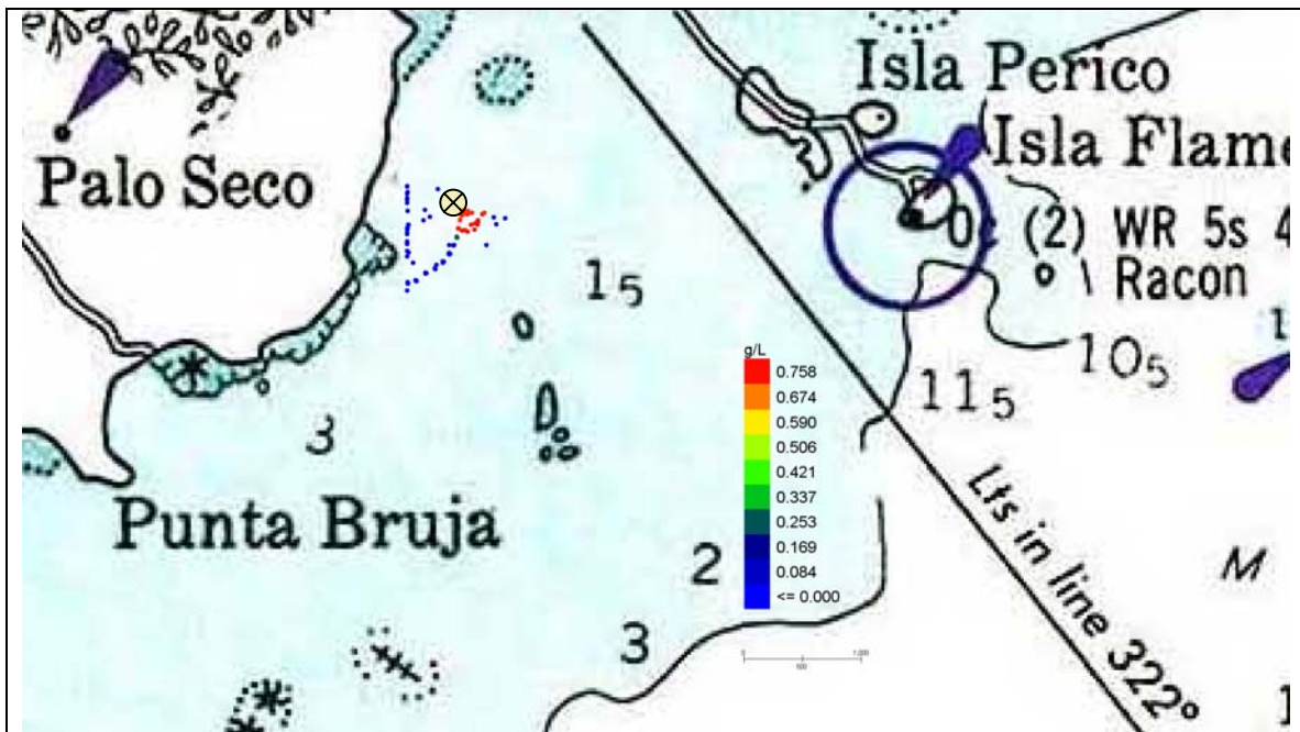
Figura 50 Escenario 4. Palo Seco. Detalle de las concentraciones de sólidos en la columna de agua a las 6 horas del comienzo del depósito.
