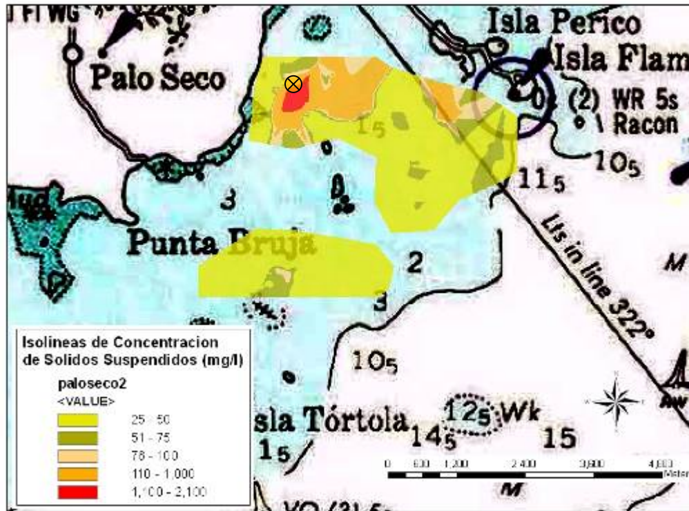
Figura 63 Escenario 4. Palo Seco. Concentraciones de sólidos en la columna de agua.
