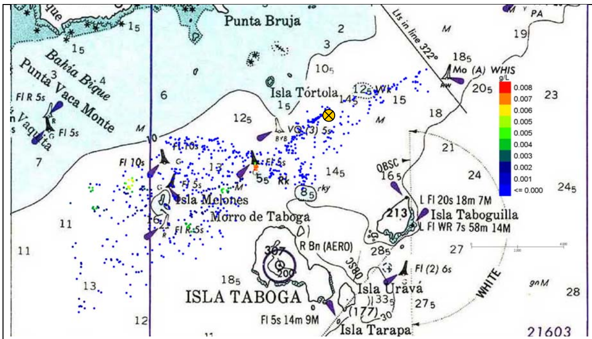
Figura 94 Escenario 7. Tortolita Sur. Detalle de las concentraciones de sólidos en la columna de agua en el día 2 (48 horas) desde el comienzo del depósito.
