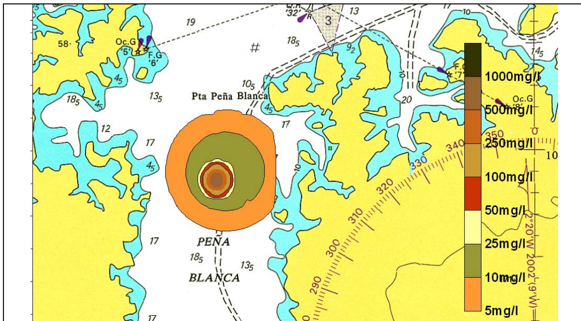
Figura 145 Escenario 11. Peña Blanca Oeste. Isolíneas de concentración a 6 m de profundidad, 9 horas después de la primera descarga.
