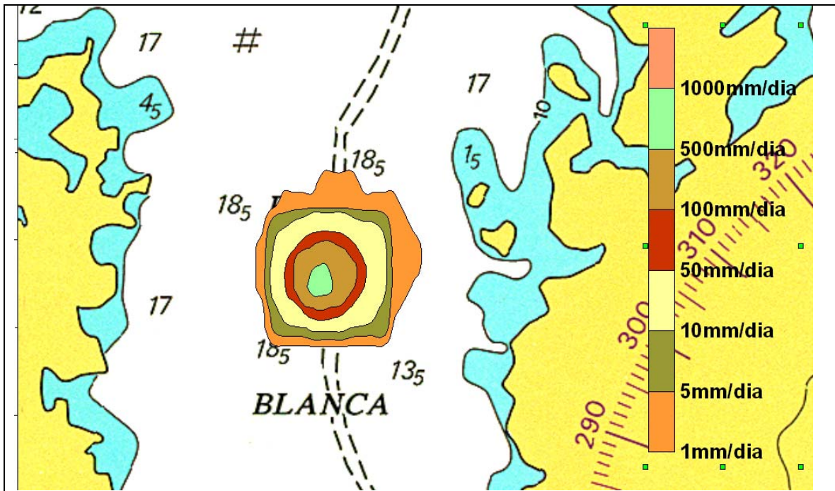
Figura 139 Escenario 11. Peña Blanca Oeste. Espesores totales de sedimentos 24 horas después de la primera descarga.
