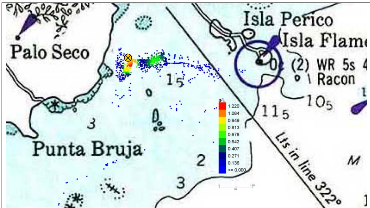
Figura 54 Escenario 4. Palo Seco. Detalle de las concentraciones de sólidos en la columna de agua en el día 2 (48 horas) desde el comienzo del depósito.
