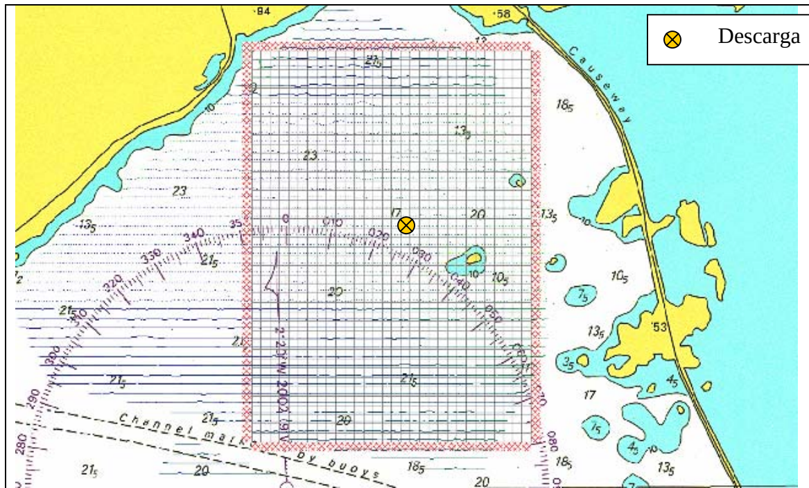
Figura 118 Malla de cálculo para la simulación de la evolución del sedimento en Monte Lirio.
