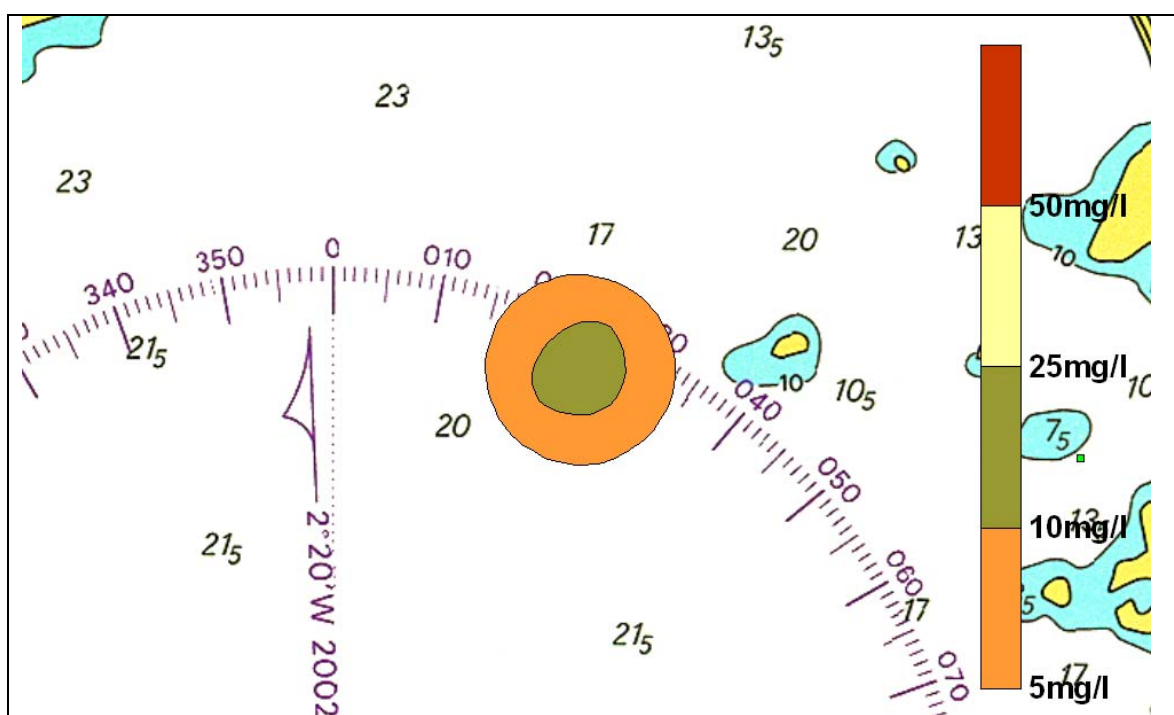
Figura 122 Escenario 9. Monte Lirio. Isolíneas de concentración a 3 m de profundidad, 4 horas después de la primera descarga.
