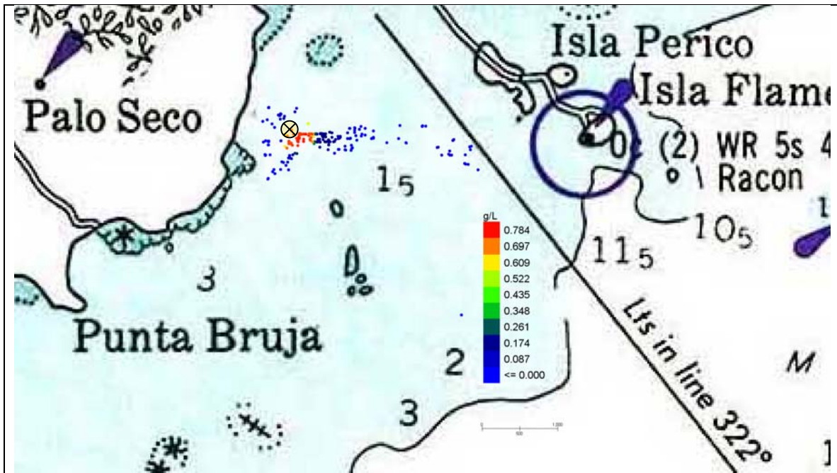
Figura 51 Escenario 4. Palo Seco. Detalle de las concentraciones de sólidos en la columna de agua a las 12 horas del comienzo del depósito.
