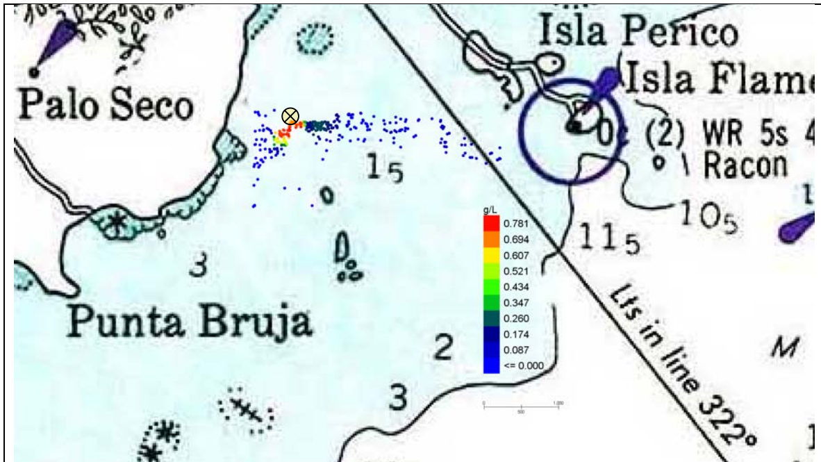
Figura 40 Escenario 3. Palo Seco. Detalle de las concentraciones de sólidos en la columna de agua a las 18 horas del comienzo del depósito.
