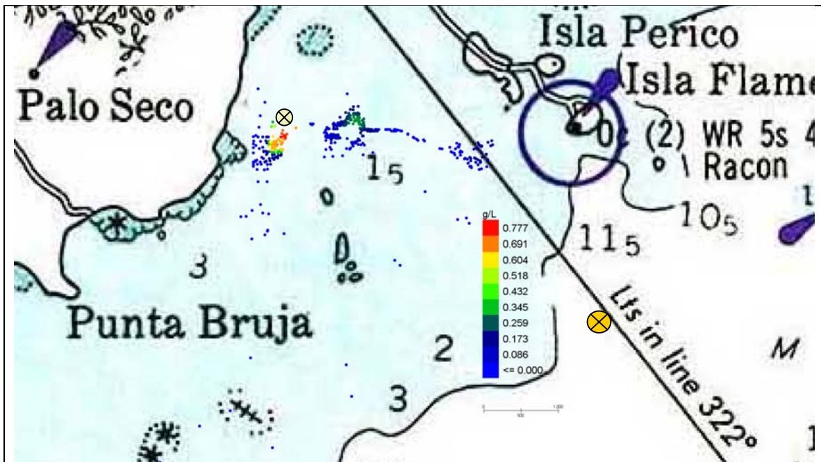
Figura 43 Escenario 3. Palo Seco. Detalle de las concentraciones de sólidos en la columna de agua en el día 3 (72 horas) desde el comienzo del depósito.
