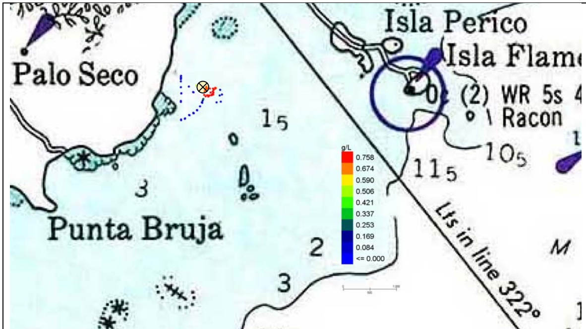
Figura 38 Escenario 3. Palo Seco. Detalle de las concentraciones de sólidos en la columna de agua a las 6 horas del comienzo del depósito.
