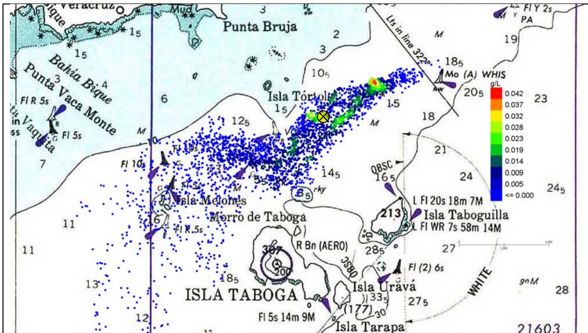
Figura 109 Escenario 8. Tortolita Sur. Detalle de las concentraciones de sólidos en la columna de agua en el día 5 (120 horas) desde el comienzo del depósito.
