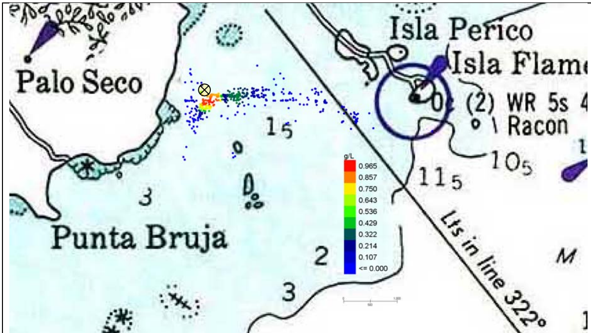
Figura 53 Escenario 4. Palo Seco. Detalle de las concentraciones de sólidos en la columna de agua en el día 1 (24 horas) desde el comienzo del depósito.
