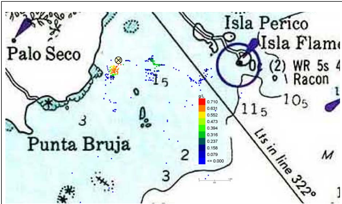
Figura 46 Escenario 3. Palo Seco. Detalle de las concentraciones de sólidos en la columna de agua en el día 6 (144 horas) desde el comienzo del depósito.
