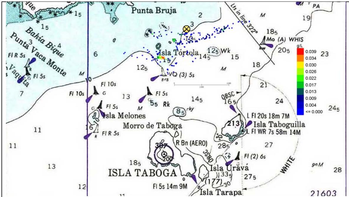
Figura 77 Escenario 6. Tortolita. Detalle de las concentraciones de sólidos en la columna de agua a las 12 horas del comienzo del depósito.
