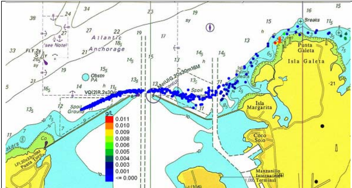
Figura 11 Escenario 1. Rompeolas Oeste. Detalle de las concentraciones de los sólidos en la columna de agua en el día 3 (72 horas) desde el comienzo del depósito.
