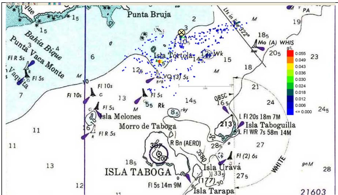
Figura 78 Escenario 6. Tortolita. Detalle de las concentraciones de sólidos en la columna de agua a las 18 horas del comienzo del depósito.
