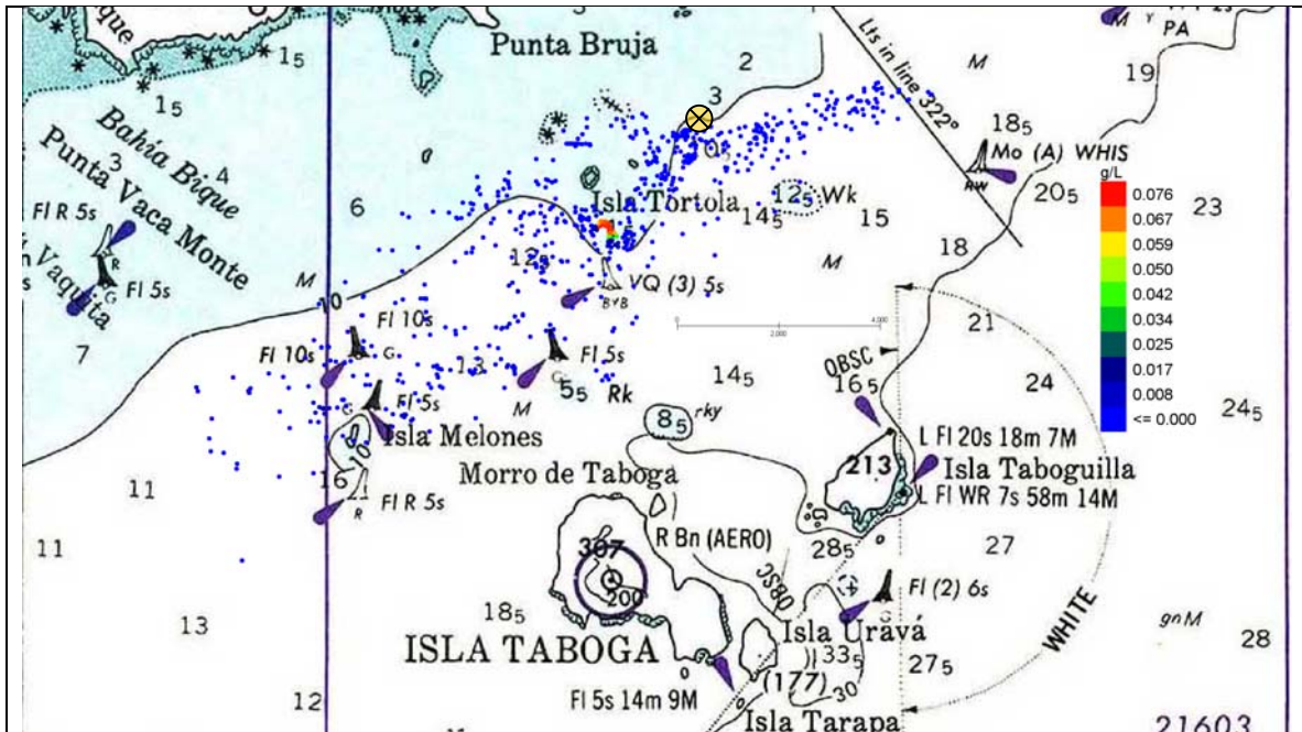
Figura 68 Escenario 5. Tortolita. Detalle de las concentraciones de sólidos en la columna de agua en el día 2 (48 horas) desde el comienzo del depósito.
