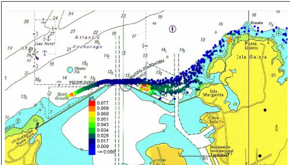
Figura 25 Escenario 2 Rompeolas Oeste. Detalle de las concentraciones de los sólidos en la columna de agua en el día 5 (120 horas) desde el comienzo del depósito.
