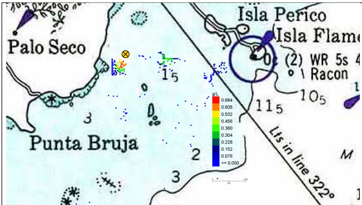
Figura 47 Escenario 3. Palo Seco. Detalle de las concentraciones de sólidos en la columna de agua en el día 7 (168 horas) desde el comienzo del depósito.
