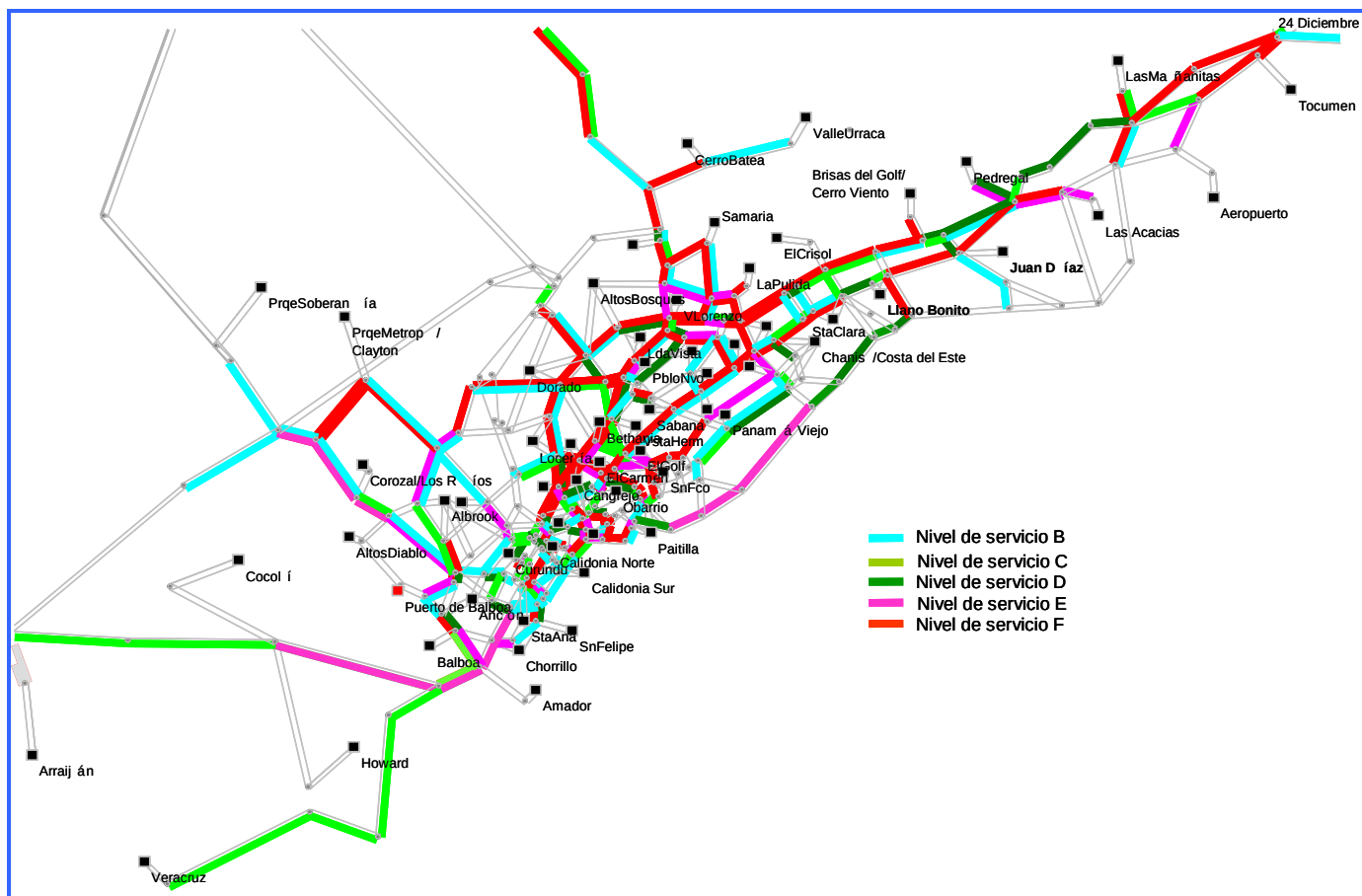
Figura 4. Niveles de Servicio en la Red Vial del Área Metropolitana del Pacífico. Año 2006 3 .
