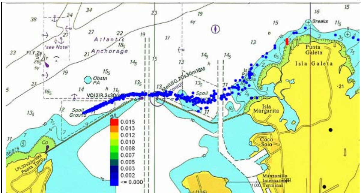
Figura 14 Escenario 1. Rompeolas Oeste. Detalle de las concentraciones de los sólidos en la columna de agua en el día 6 (144 horas) desde el comienzo del depósito
