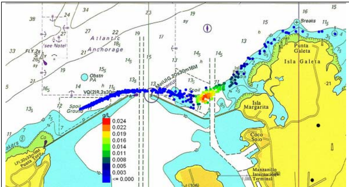
Figura 10 Escenario 1. Rompeolas Oeste. Detalle de las concentraciones de los sólidos en la columna de agua en el día 2 (48 horas) desde el comienzo del depósito.
