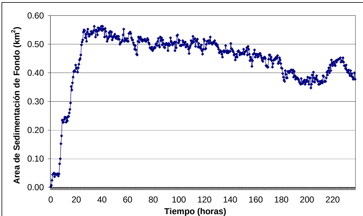
Figura 48 Escenario 3. Palo Seco. Evolución temporal de las áreas de fondo donde el espesor de sólidos depositados es superior a 0.1 mm.
