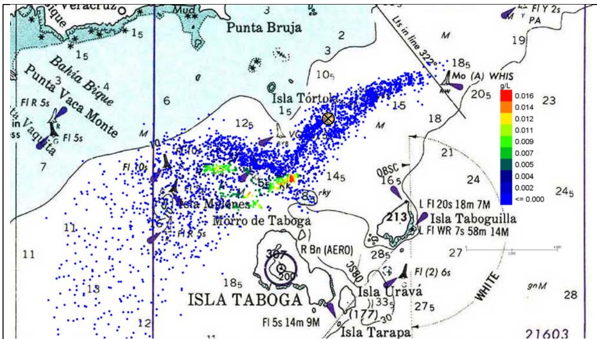
Figura 111 Escenario 8. Tortolita Sur. Detalle de las concentraciones de sólidos en la columna de agua en el día 7 (168 horas) desde el comienzo del depósito.
