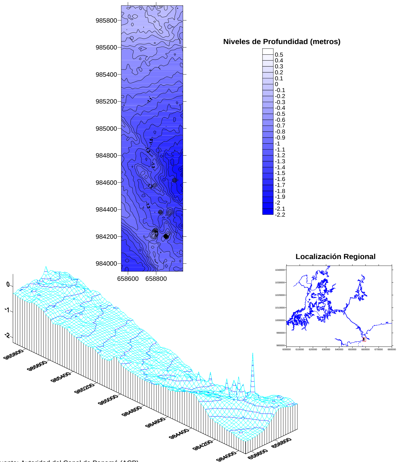
Figura N°4-10 Batimetría del Sitio de Depósito Palo Seco (Agosto de 2006)
