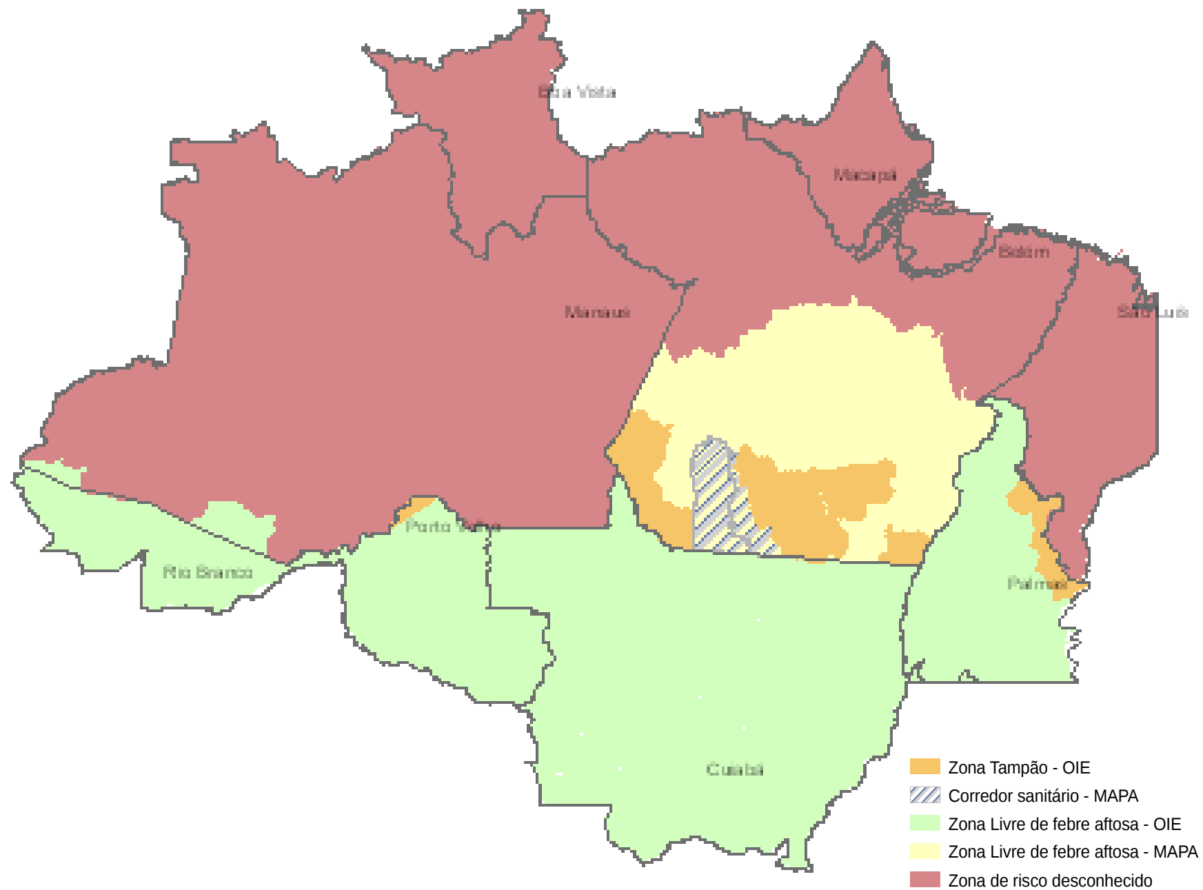
Figura 2. Classificação das zonas de risco de febre aftosa na Amazônia Legal
